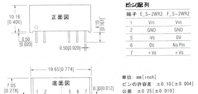
外觀図 LxWxH: 19.65x7.05x10.16(mm)
