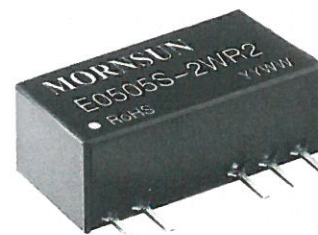
外觀図 LxWxH: 19.65x7.05x10.16(mm)
