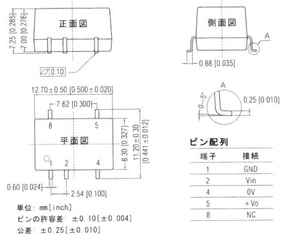
外觀図 LxWxH: 12.70x11.20x7.25(mm)
